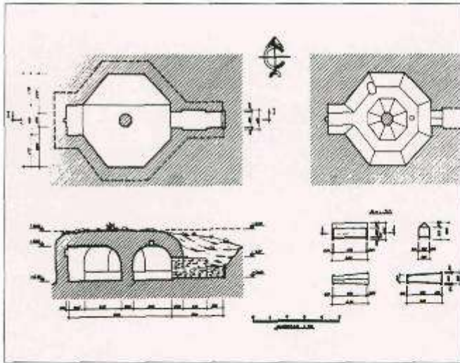
Xarabagilan sərdabəsinin sxematik planı.
